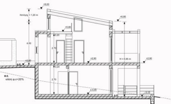
ΚΤΙΠΙΟ 3 - ΤΟΜΗ Α-Α
